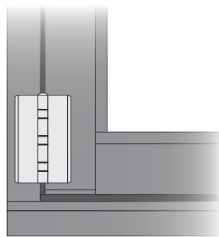
Narrow G3 Jamb & Standard G3 Frame
