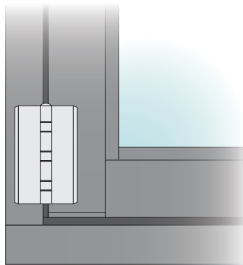
Narrow G2 Jamb & Regular G2 Frame
