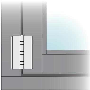
Regular G2 Jamb & Frame
